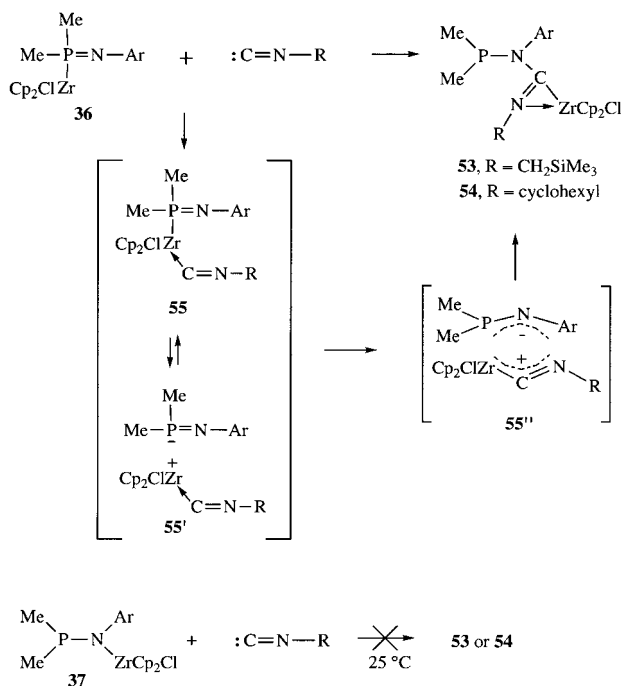
Scheme 14.
